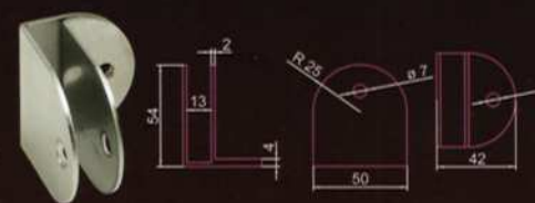
Soporte sujeción / escuadra ref. 592
