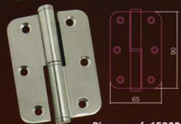
Bisagra ref. 6590D (Derecha) 6590I (Izquierda)
